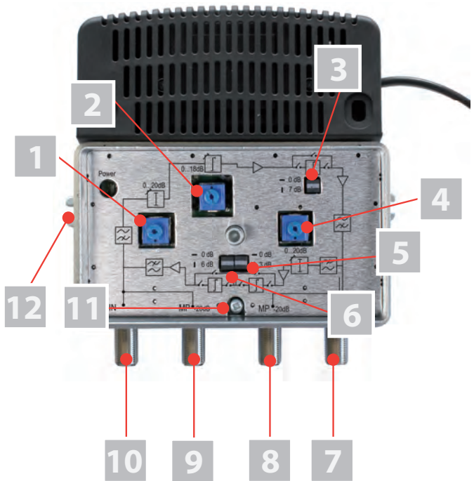
Bild 2: Verstärker HVC 42, Innenansicht
